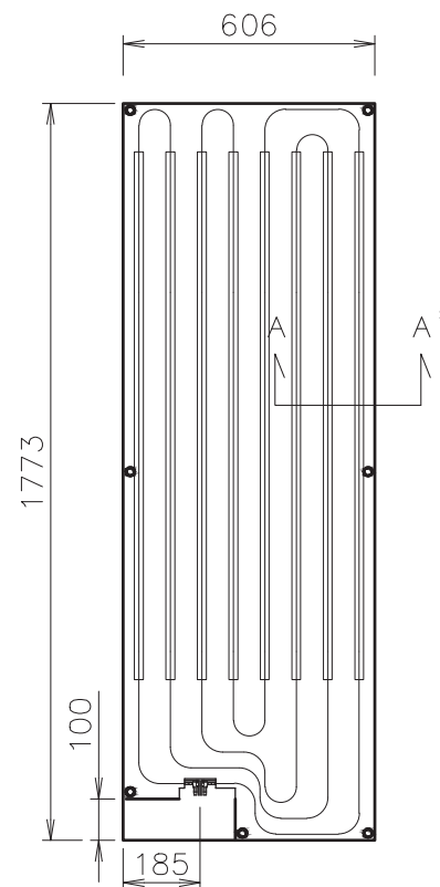
ヘッダー部詳細図
