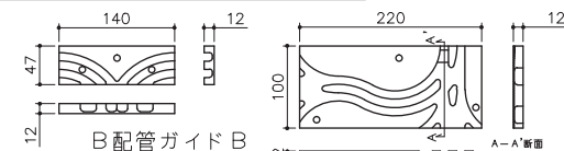
B 配管ガイド A L
