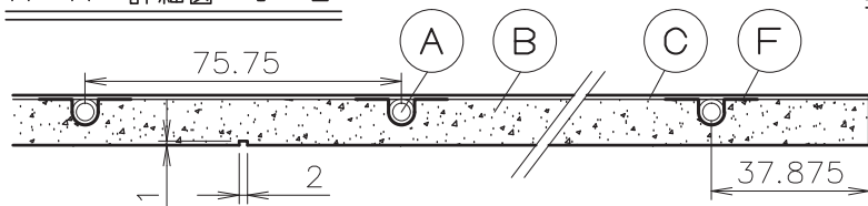
A-A' 詳細図 1 / 2
