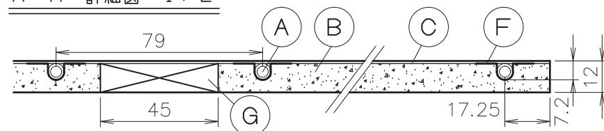
A-A' 詳細図 1/2
