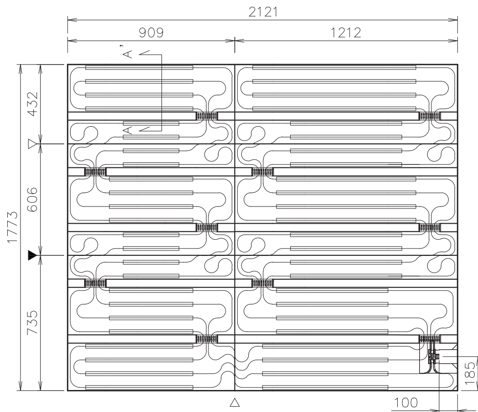
ヘッダー部詳細図
