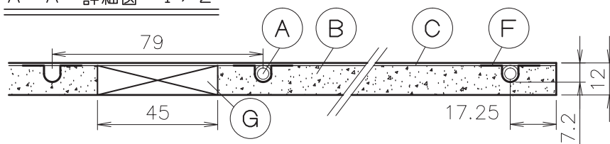
A-A' 詳細図 1 / 2
