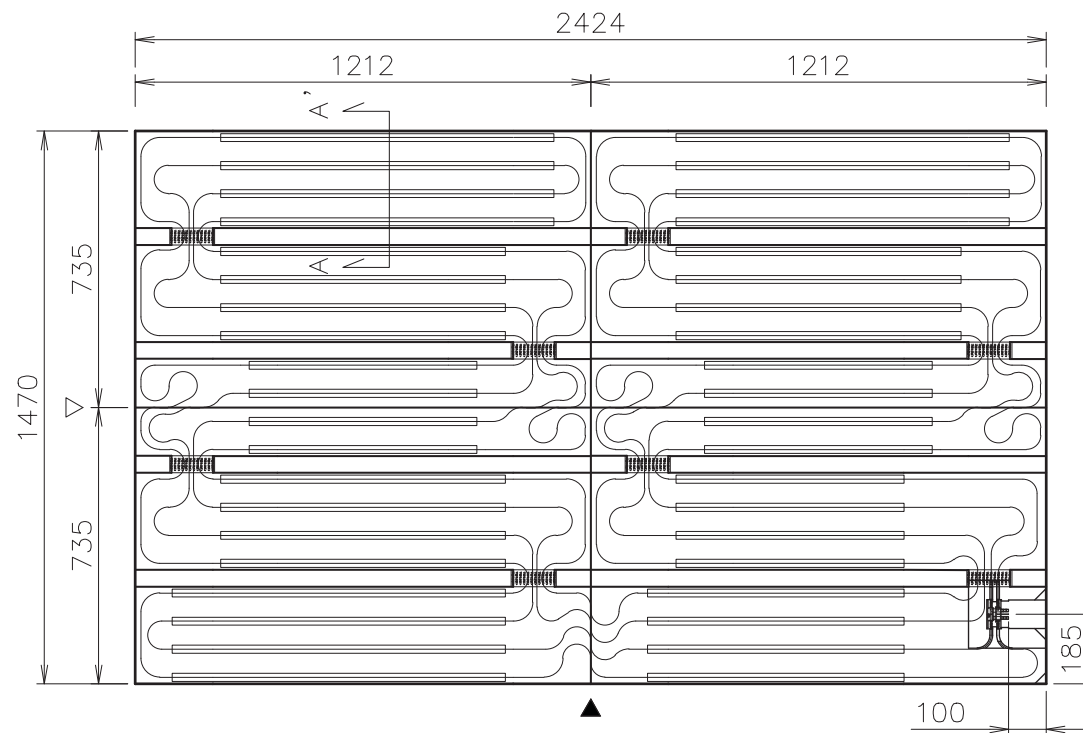
ヘッダー部詳細図
