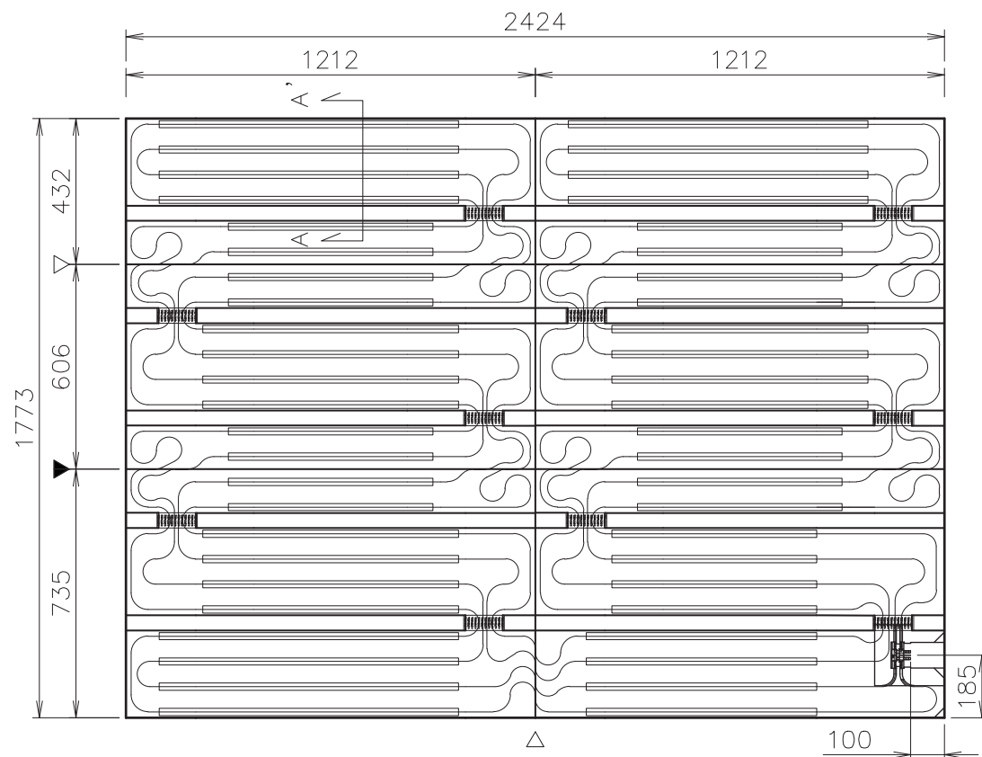
ヘッダー部詳細図
