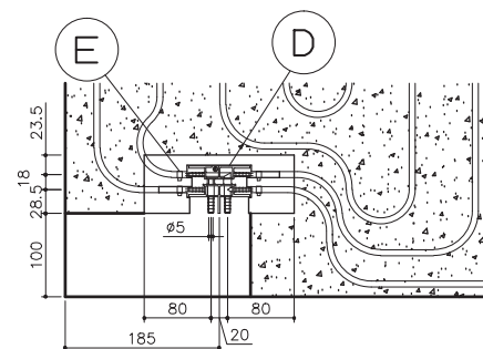
ヘッダー部詳細図
