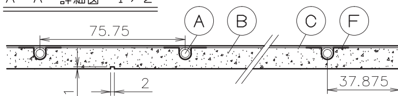
A - A' 詳細図 1 / 2
