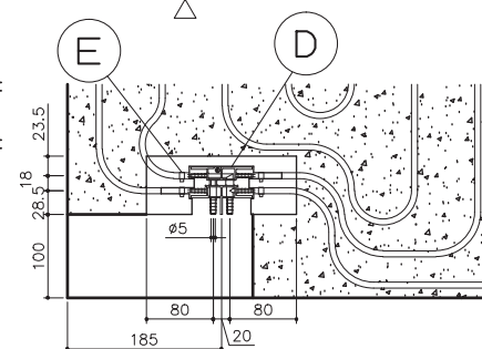
ヘッダー部詳細図 1 / 10
