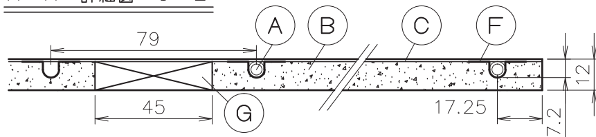
A-A' 詳細図 1 / 2
