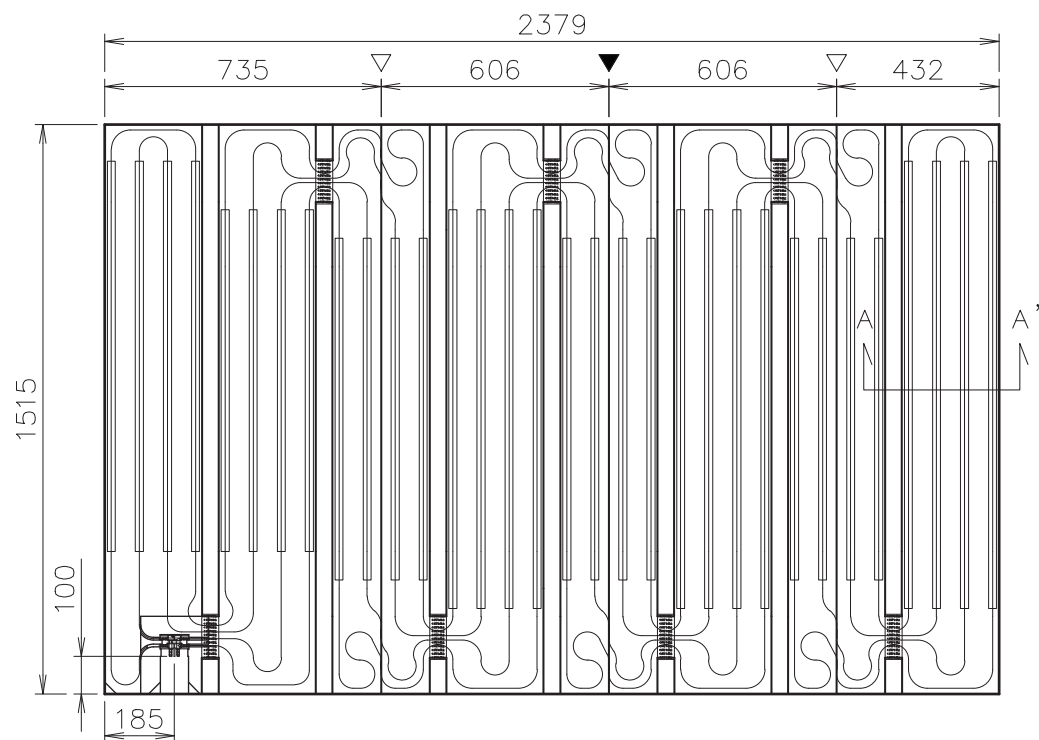
ヘッダー部詳細図
