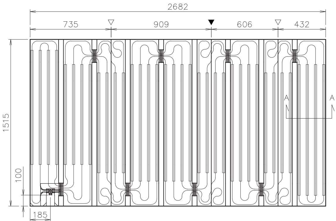
ヘッダー部詳細図
