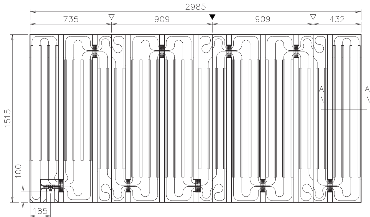
ヘッダー部詳細図
