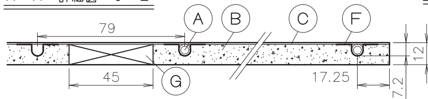
A-A' 詳細図 1/2
