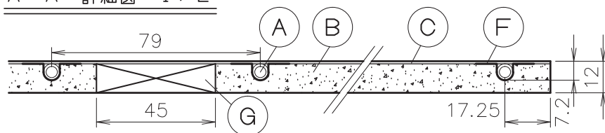
A-A' 詳細図 1 / 2
