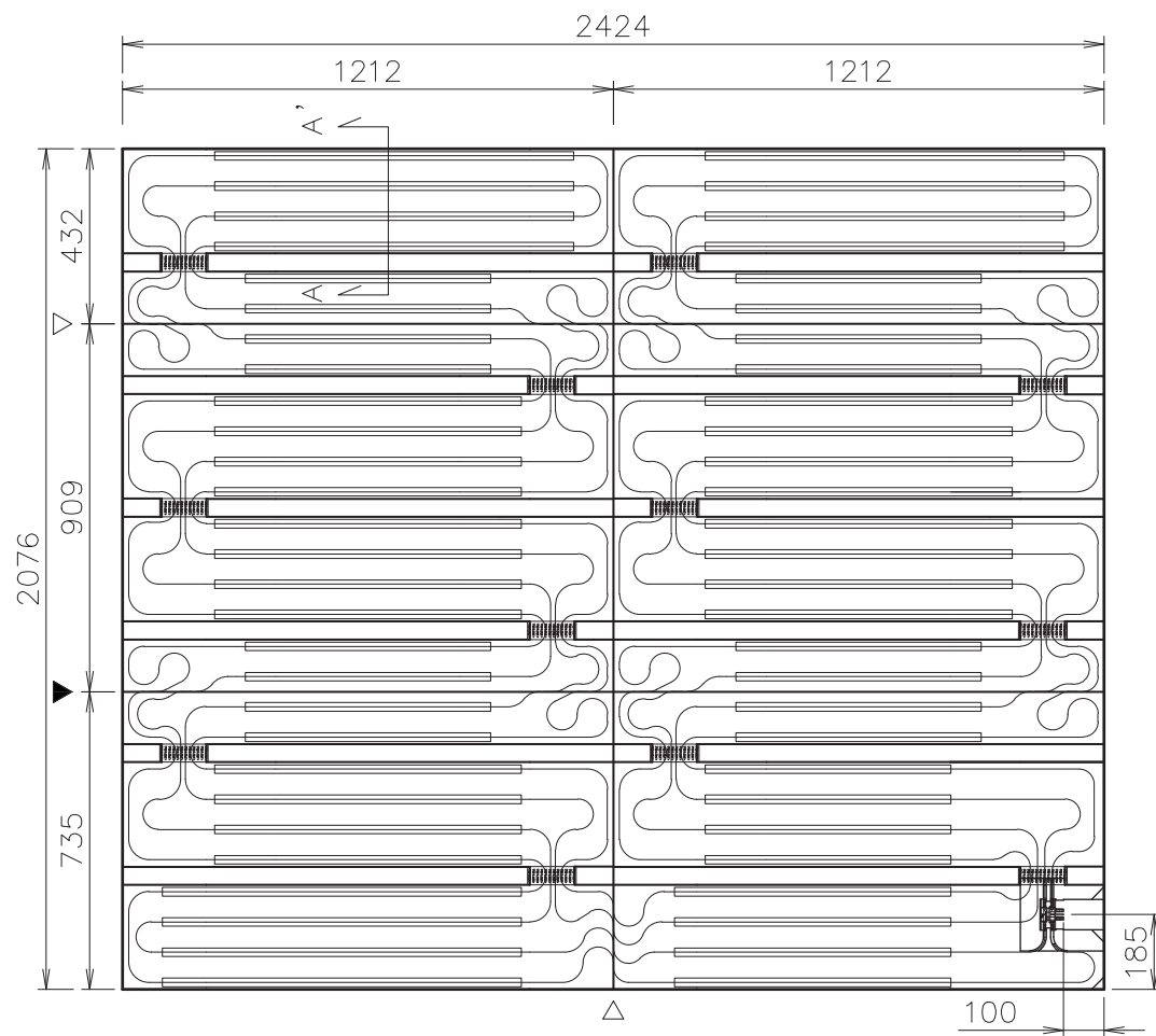
ヘッダー部詳細図
