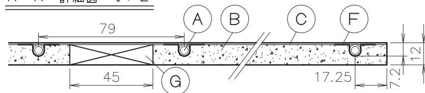
A-A' 詳細図 1/2
