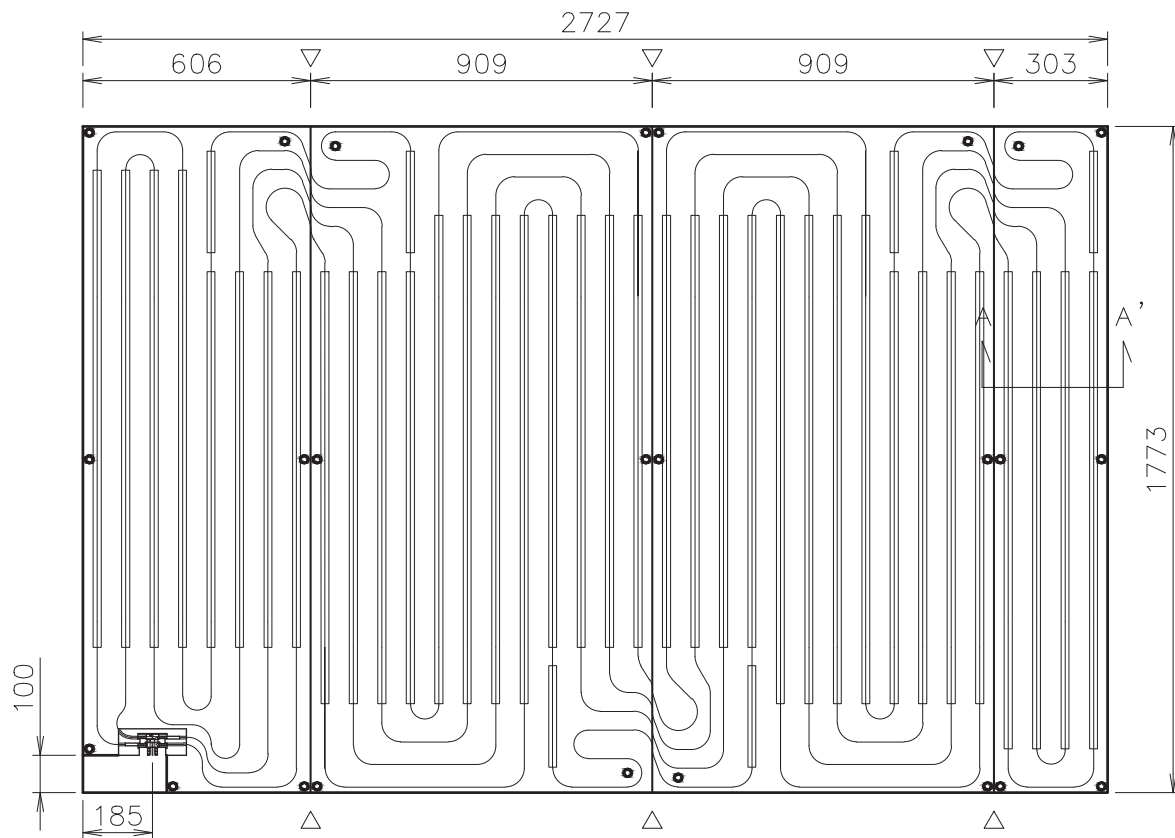
ヘッダー部詳細図
