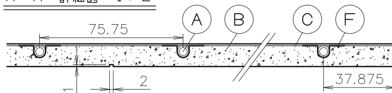
A-A' 詳細図 1 / 2
