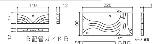
配管ガイド詳細図 1 / 10
