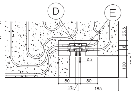
ヘッダー部詳細図
