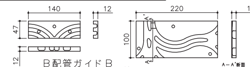
配管ガイド詳細図 1/10
