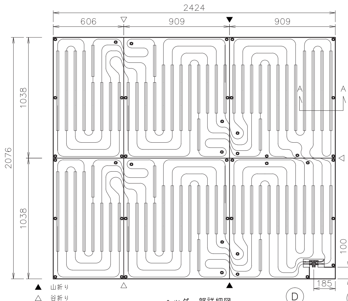
ヘッダー部詳細図
