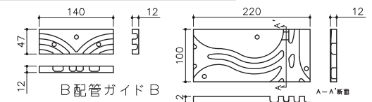
配管ガイド詳細図 1/10
