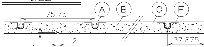
A - A' 詳細図 1 / 2
