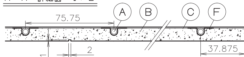
A-A' 詳細図 1 / 2
