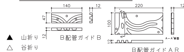
配管ガイド詳細図 1 / 10
