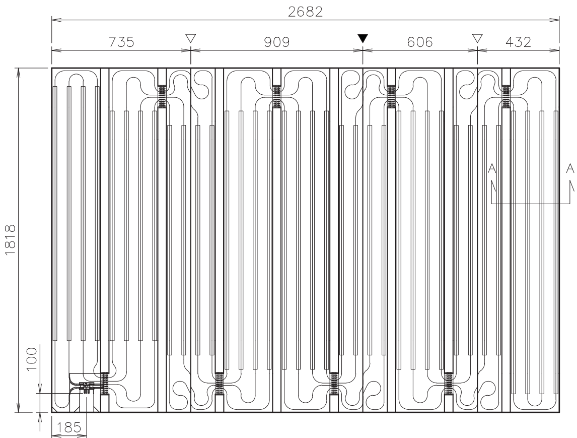
ヘッダー部詳細図
