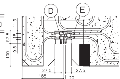
ヘッダー部詳細図
