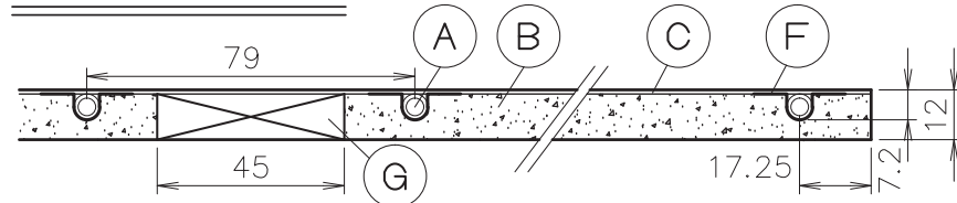
A-A' 詳細図 1/2
