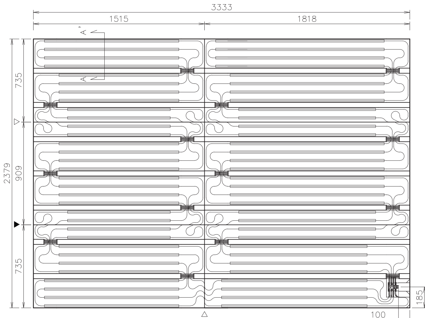
ヘッダー部詳細図
