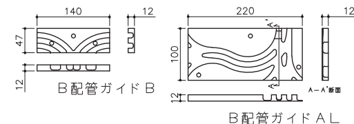
配管ガイド詳細図 1/10
