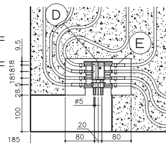
ヘッダー部詳細図
