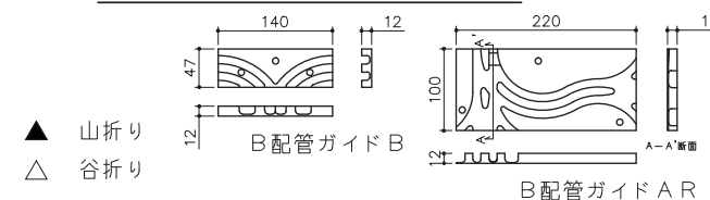
配管ガイド詳細図 1 / 10
