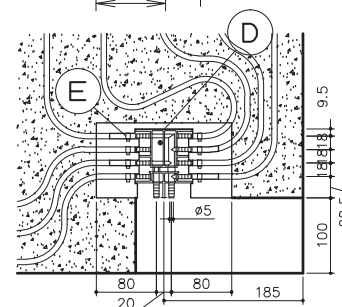
ヘッダー部詳細図
