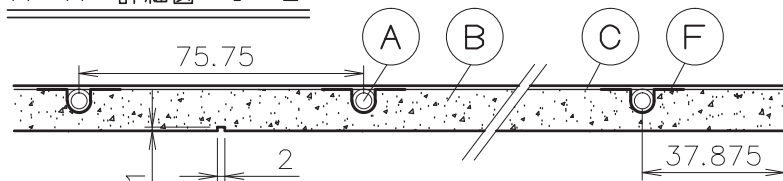
A-A' 詳細図 1 / 2
