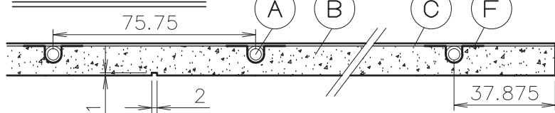
A-A' 詳細図 1 / 2
