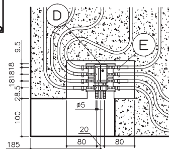
ヘッダー部詳細図 1 / 10
