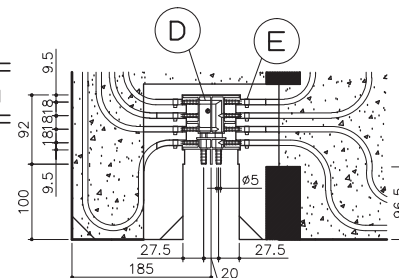
ヘッダー部詳細図
