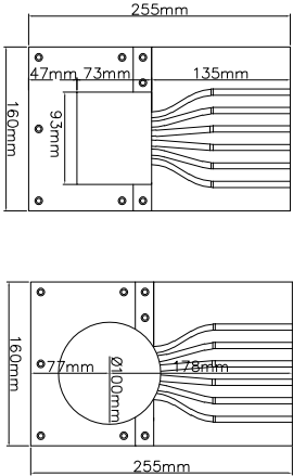
□穴開口部寸法 ○穴開口部寸法
