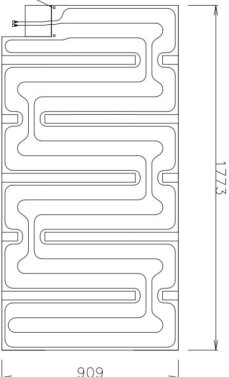
くぎ打ち検知 信号線設置 位置表示
