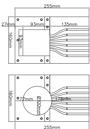
□穴開口部寸法 ○穴開口部寸法
