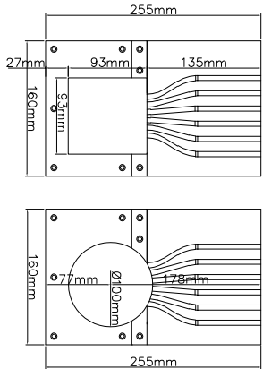
□穴開口部寸法 ○穴開口部寸法
