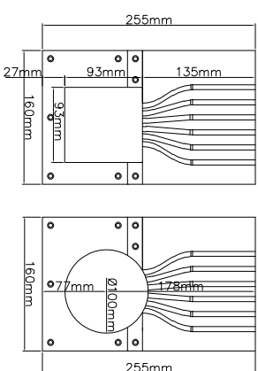
口穴開口部寸法 ○穴開口部寸法
