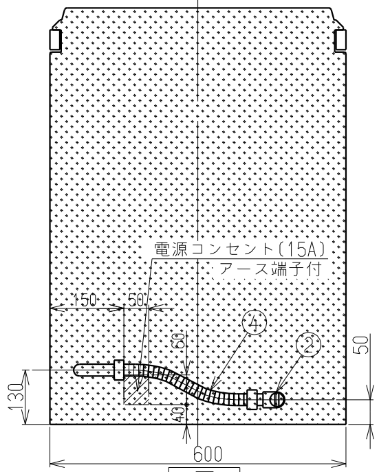
正面図
