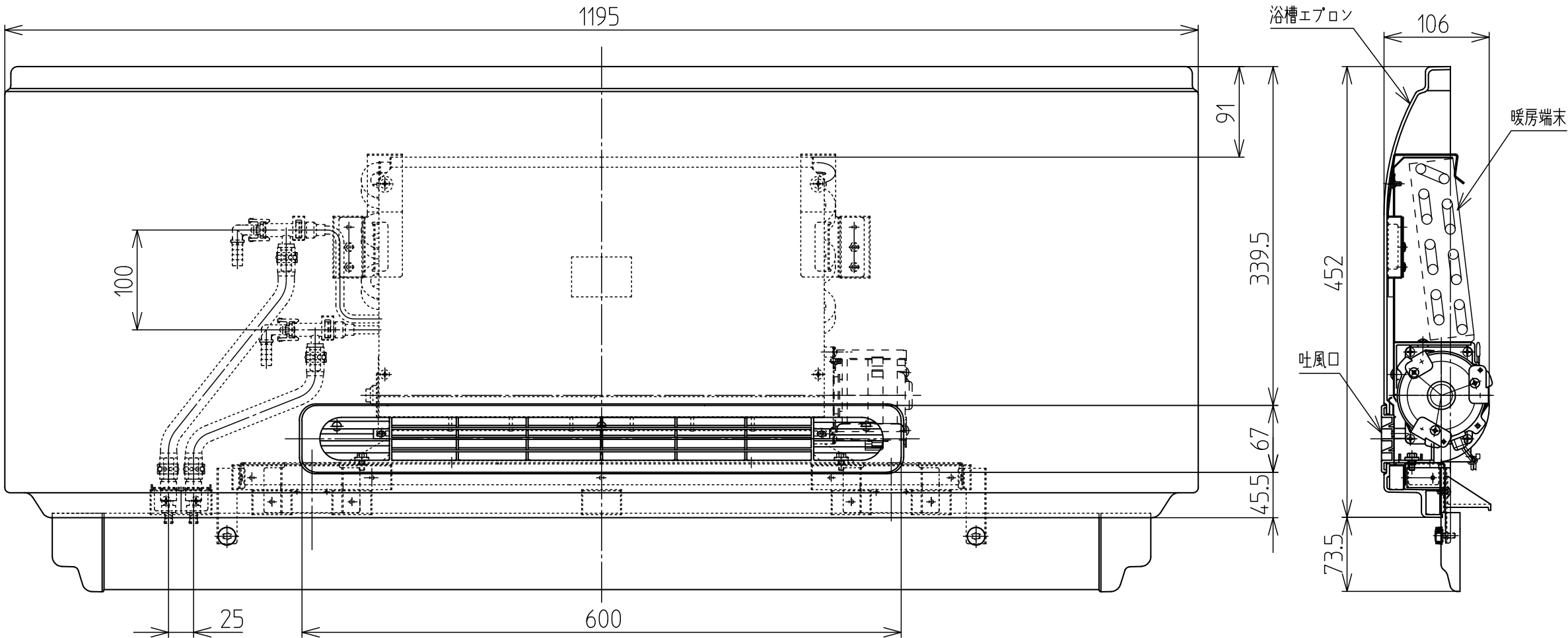
※本図は、エプロンに組み込み、アジャストカバーを取付けた状態です。
