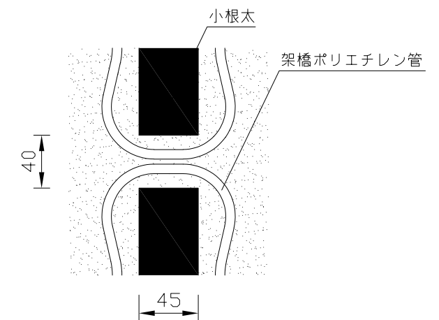
〈小根太ー小根太間拡大図〉
