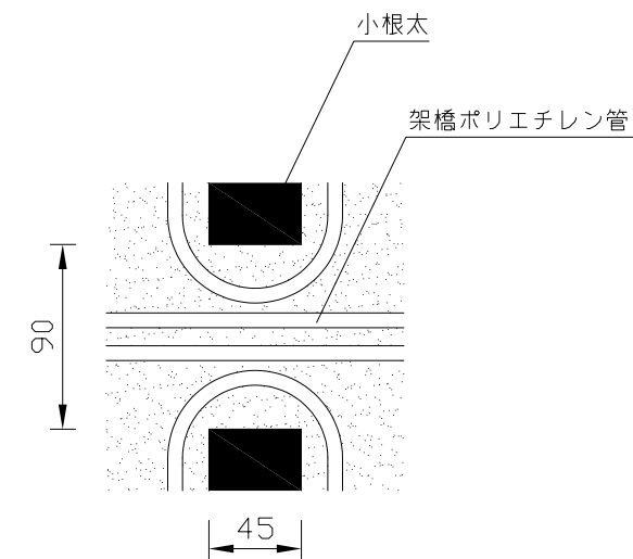
(小根太-小根太間拡大図)
