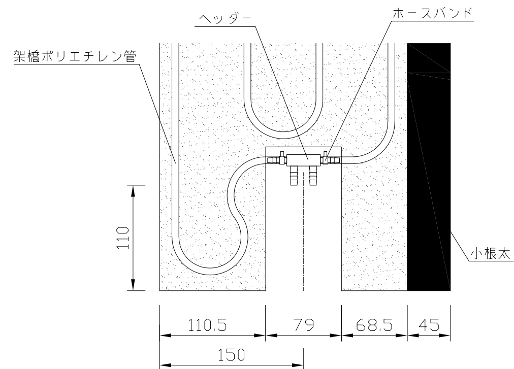
(ヘッダー部拡大図)
