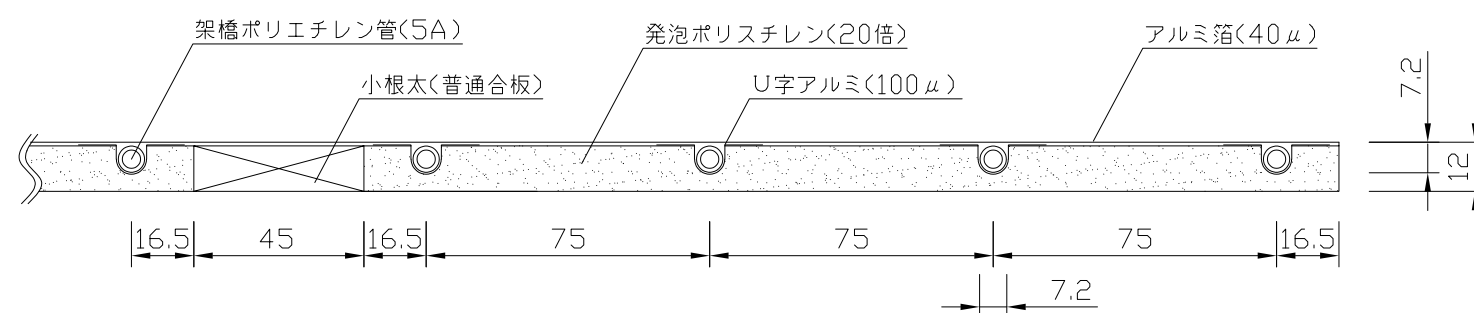
(A-A'断面図)
