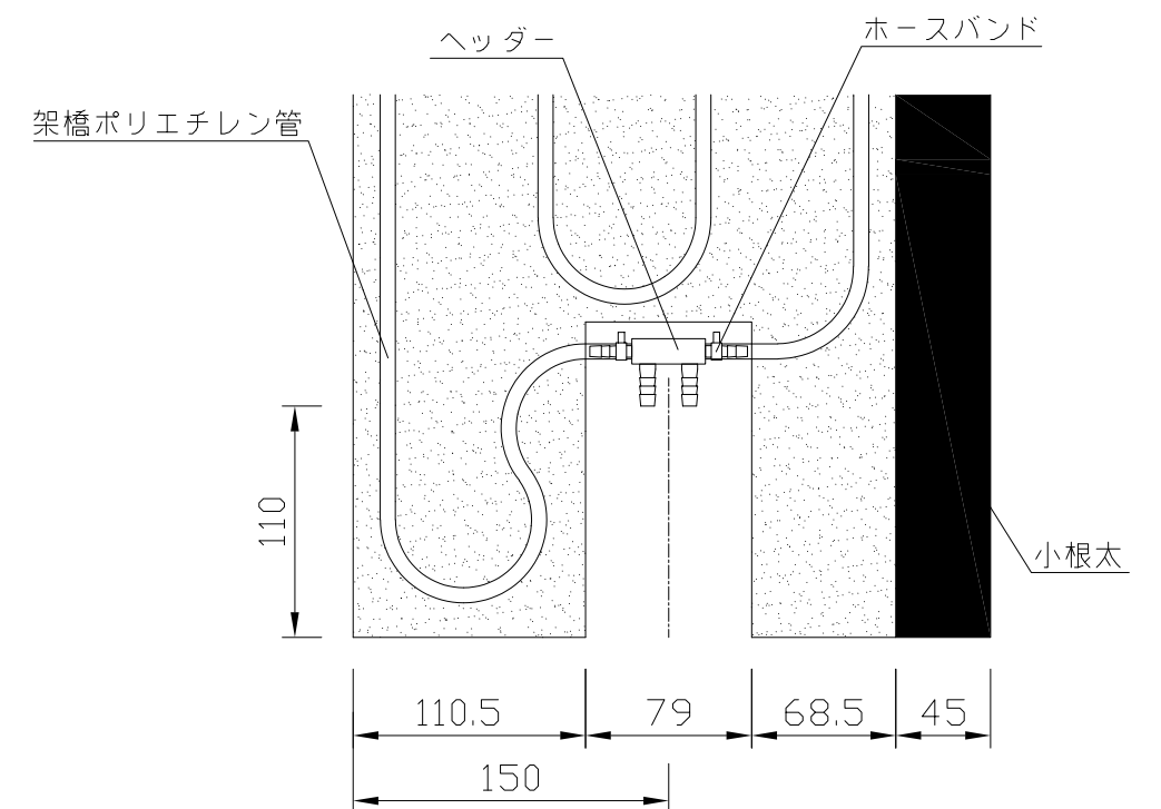
(ヘッダー部拡大図)
