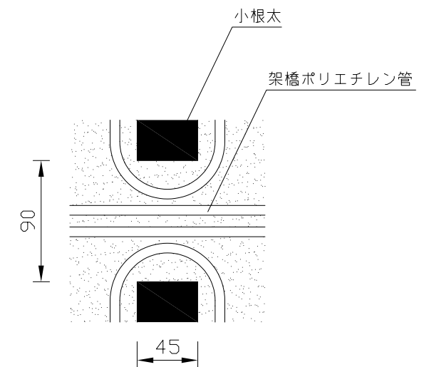
(小根太ー小根太間拡大図)
