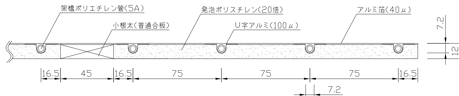
(A-A'断面図)
