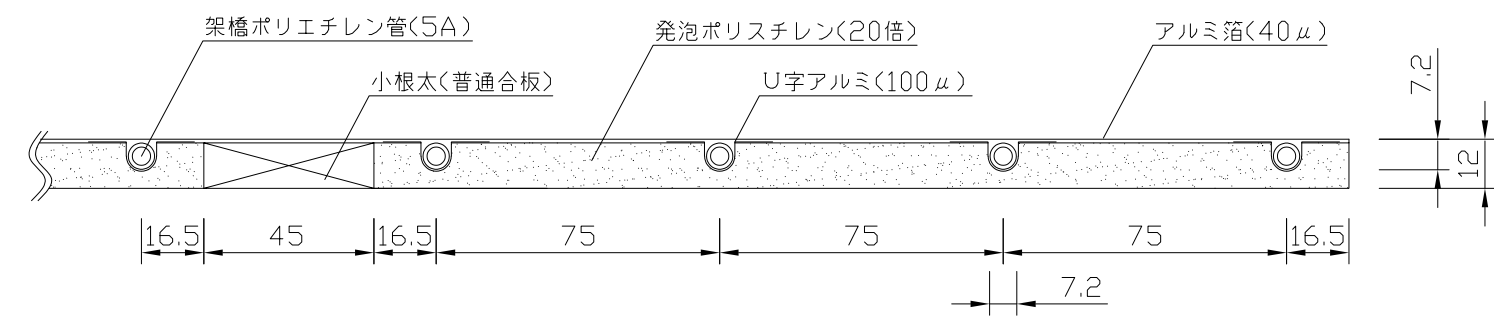
(A-A'断面図)
