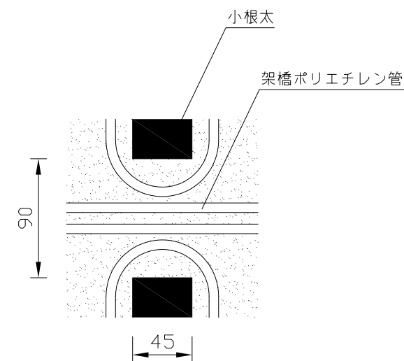
〈小根太－小根太間拡大図〉
