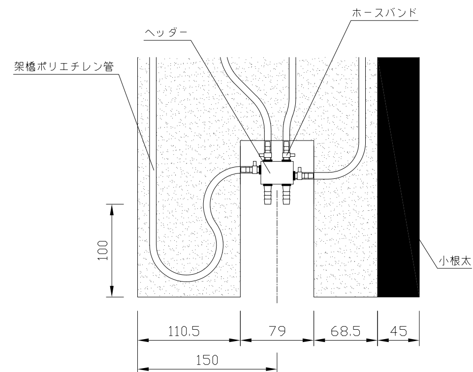
〈ヘッダー部拡大図〉
