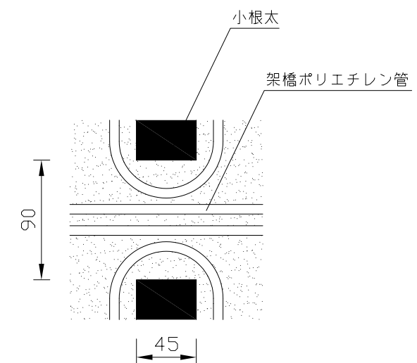
(小根太ー小根太間拡大図)
