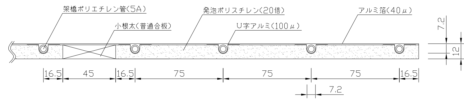
(A-A'断面図)
