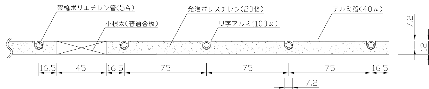
(A-A'断面図)
