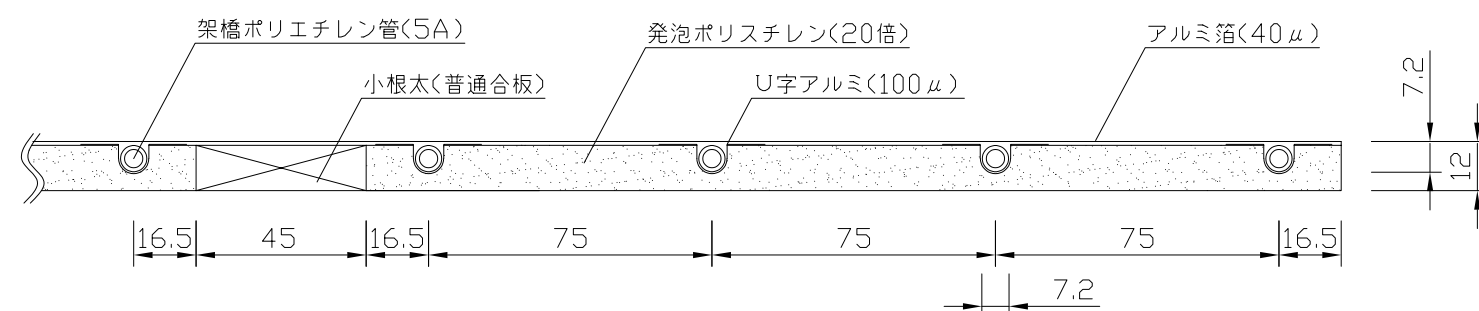
(A-A'断面図)
